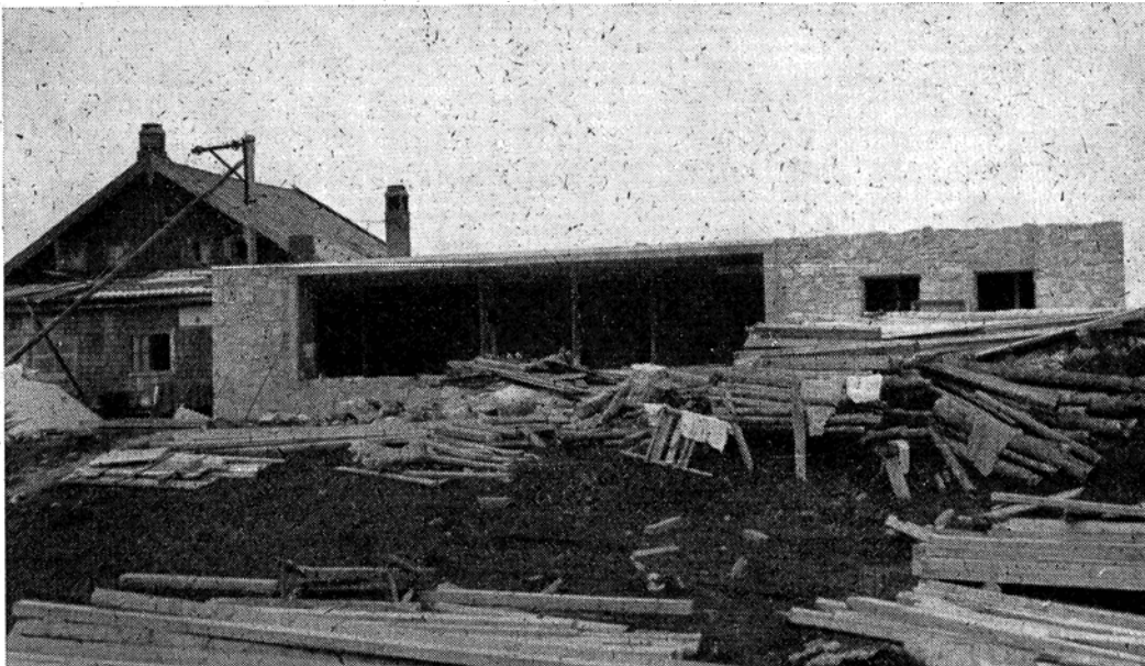
Stand des Hüttenneubaues Ende Juli 1959
